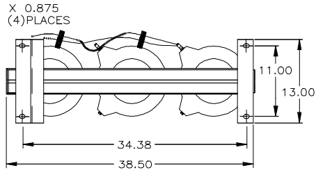
Dimensions for 60kV BIL units
