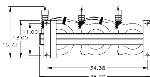
Dimensions for 95kV BIL units
