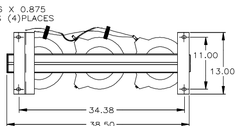
Dimensions for 60kV BIL units
