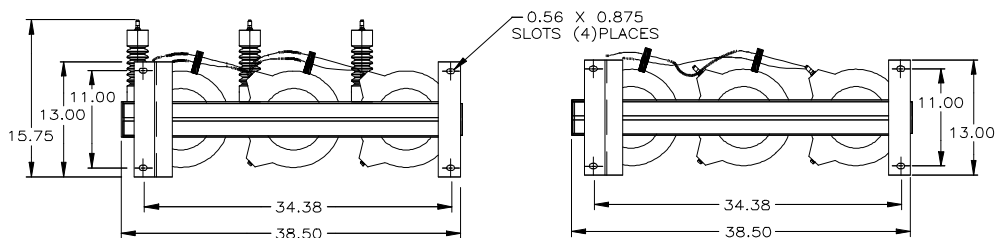
Dimensions for 95kV BIL units
